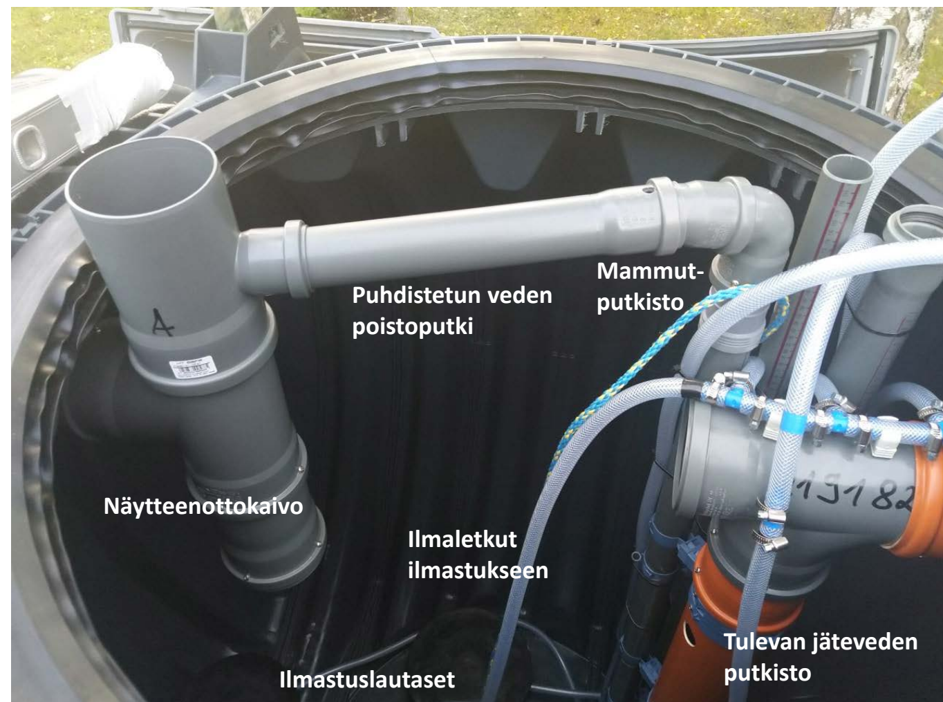
Säiliön sisäpuolinen lietekeräys
